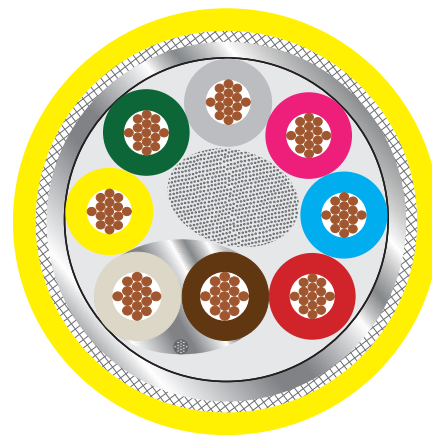
KWLI-2Y(St+C)11Y 1x2x0,5PiMF+3x2x0,5
