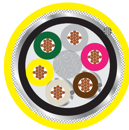
SSL2H(St+C)11Y 2x0,5AiMF+4x0,5mm 2
